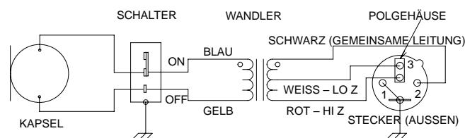
INTERNE ANSCHLÜSSE ABILDUNG 5
