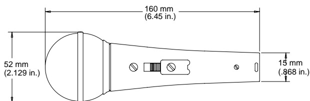
ABMESSUNGEN ABILDUNG 3
