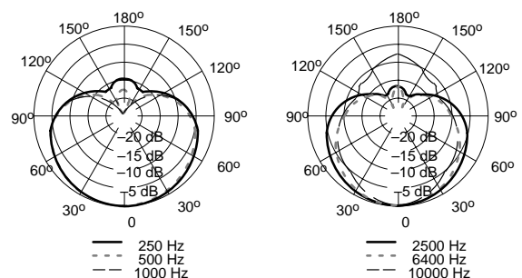
PATRONES DE CAPTACION POLAR TIPICOS FIGURA 2
