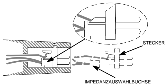
IMPEDANZAUSWAHL STECKERENDE DES MIKROPHONS ABILDUNG 4
